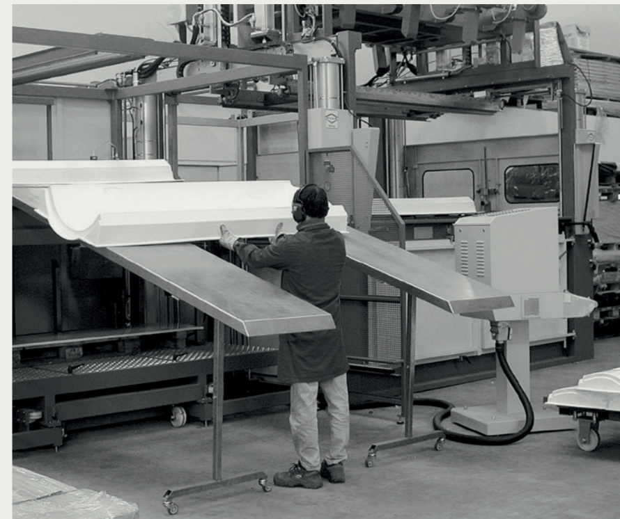
Impianto di termoformatura per materiali acrilici Thermoforming plant for acrylic materials
