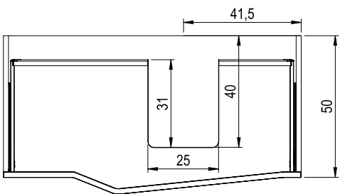
Façonnage tiroir éléments bas STR8 2 Legrabox avec collier en métal VERS GAUCHE
