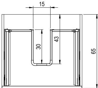
Façonnage tiroir élément bas Store P. 65 avec collier en plastique
