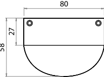
Vue de haut Вид сверху
