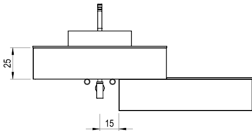
Lavabo a poser Элемент баз inférieur avec siphon à l'extérieur
