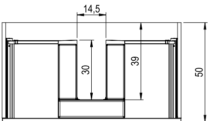
Façonnage tiroir éléments bas P. 50 avec Cuvettes en plastique (Change)
