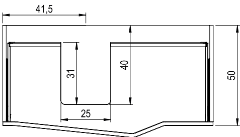
Façonnage tiroir éléments bas STR8 2 Legrabox avec collier en métal VERS DROITE
