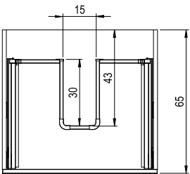
Fond du meuble avec découpe pour siphon en plastique (voir page 23) Дном с внутренним вырезом под сифон из пластика (см. стр. 23)
