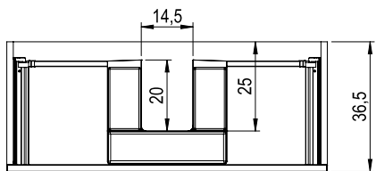
Façonnage tiroir éléments bas P. 36,5 avec Cuvettes en plastique (Change)
