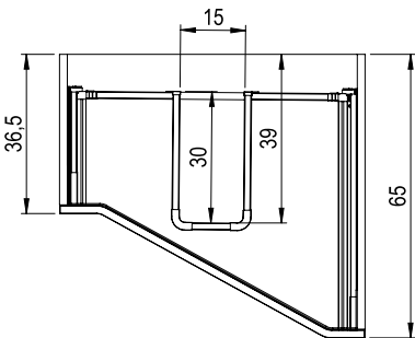
Façonnage tiroir élément bas Store Excellent avec collier en plastique
