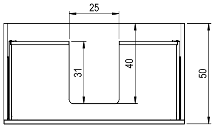
Façonnage tiroir éléments bas P. 50 Legrabox avec collier en métal
