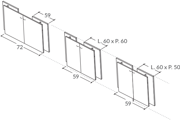
Mobile pieghevole per lavatoio in ceramica Folding cabinet for ceramic sink
