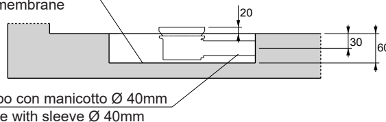
S2: SCARICO PIATTO DOCCIA / SHOWER DRAIN
